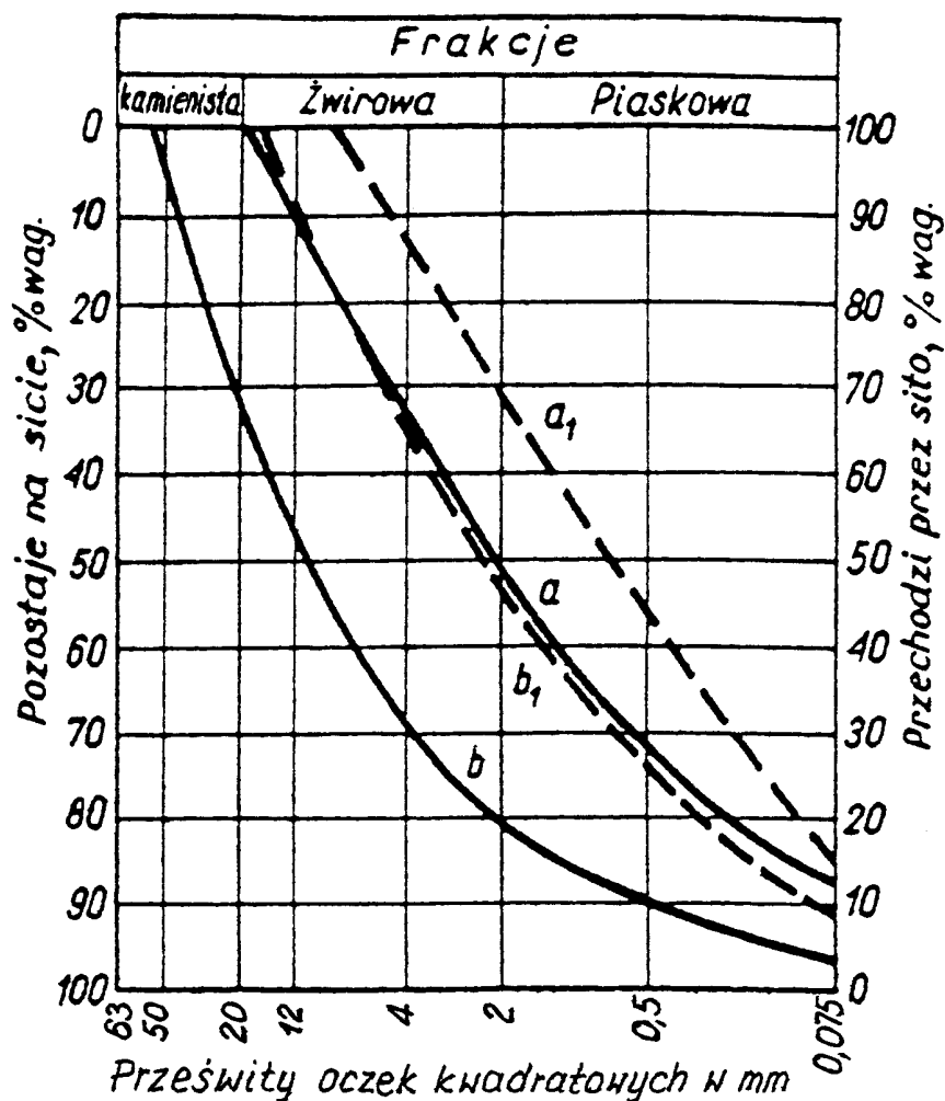
Rysunek 1. Obszar uziarnienia optymalnych mieszanki żwirowych
